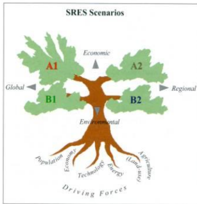
Figure 31. SRES Scenarios.
